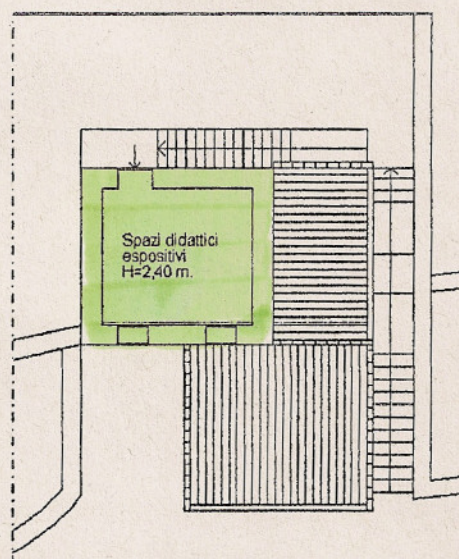
Piano secondo
